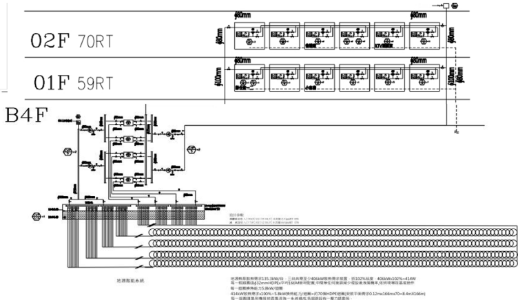
將捷之森空調架構圖
